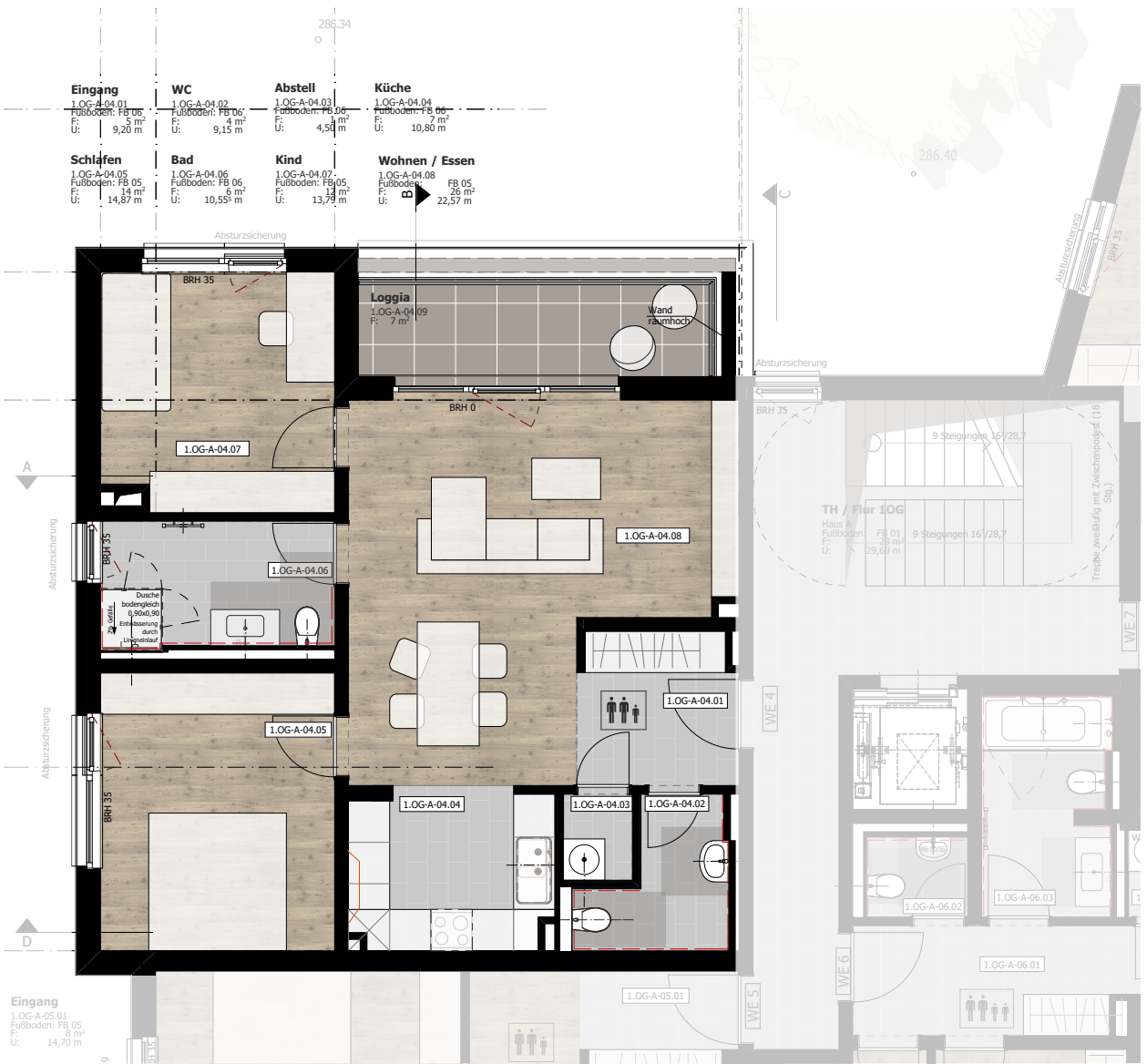
Haus A - Wohnung 04 1. Obergeschoss | 1:100
