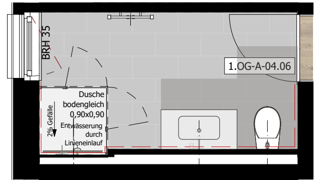
Haus A - Wohnung 04 - Bad 1. Obergeschoss | 1:50
