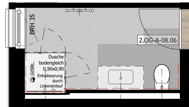
Haus A - Wohnung 08 - Bad 2. Obergeschoss | 1:50
