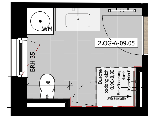
Haus A - Wohnung 09 - Bad 2. Obergeschoss | 1:50
