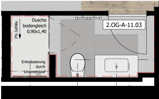
Haus A - Wohnung 11 - Bad 2. Obergeschoss | 1:50
